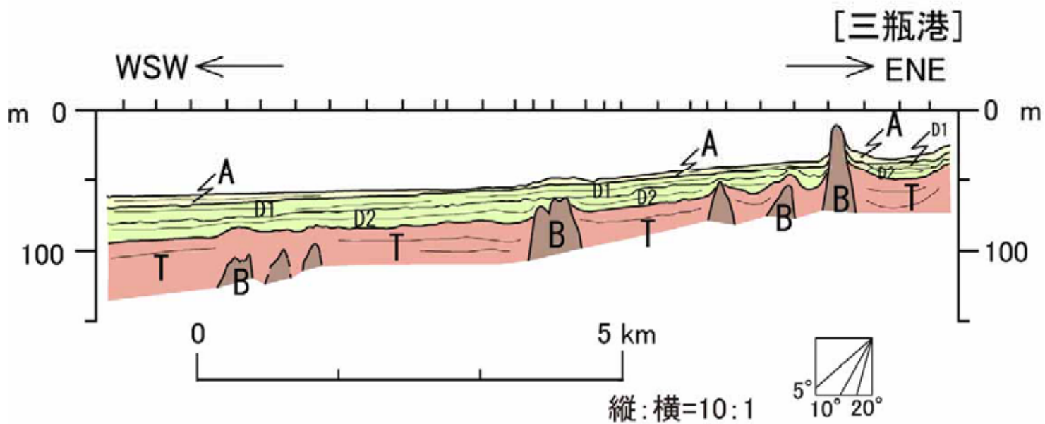
図-93 F-21 断層東方延長部の海底地質断面図②
