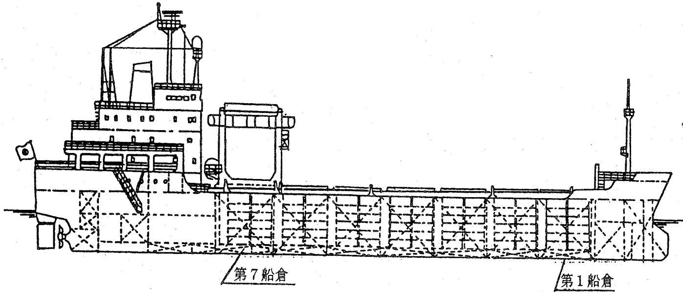
側面図
