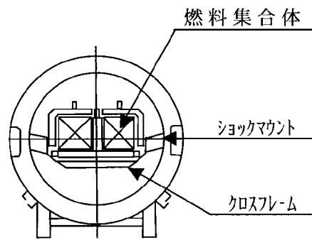
断面A-A
