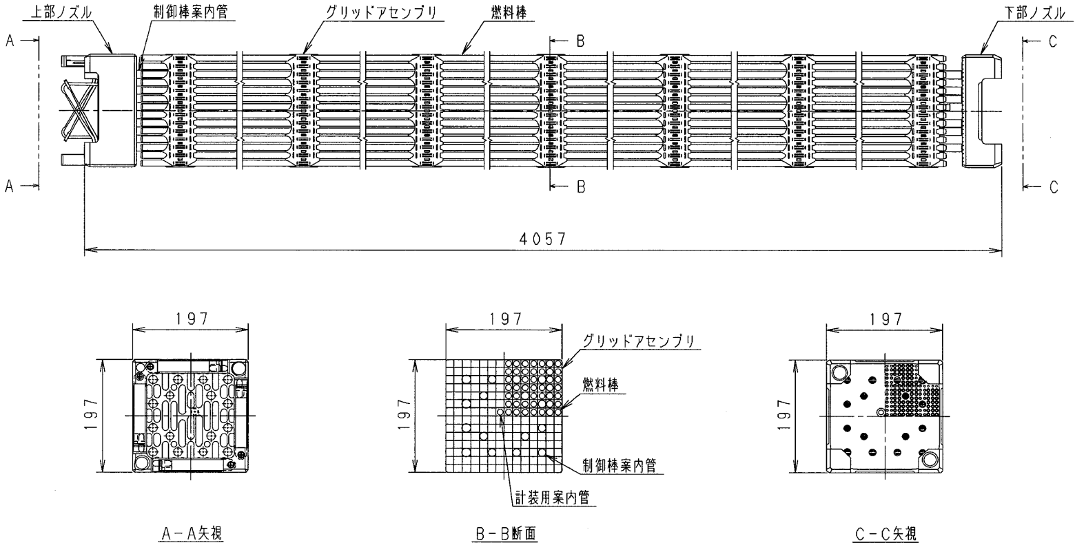
図1 燃料集合体（1号機用）（1/3）
