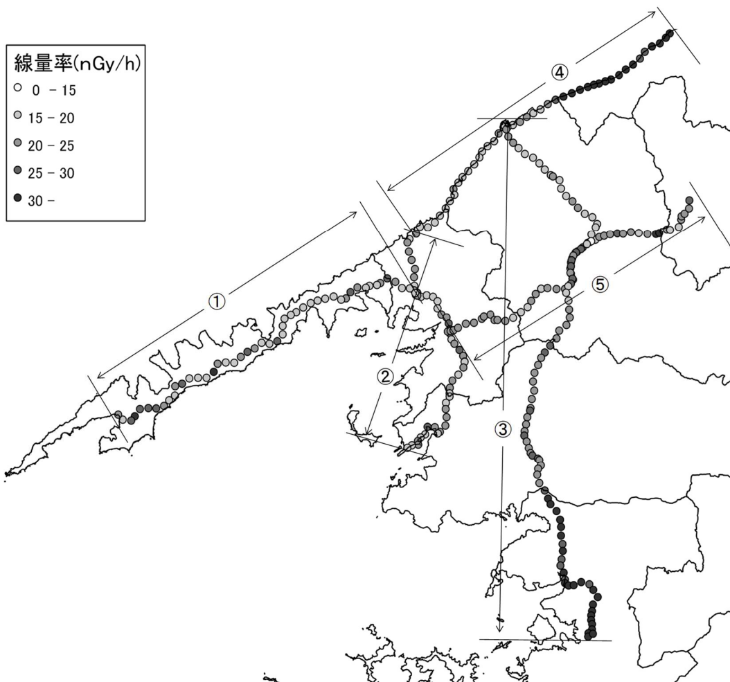
図2-1 3"φ×3"NaI (T1) シンチレーション検出器 (温度補償・エネルギー補償回路付) による測定結果 (地図上データ表示)
