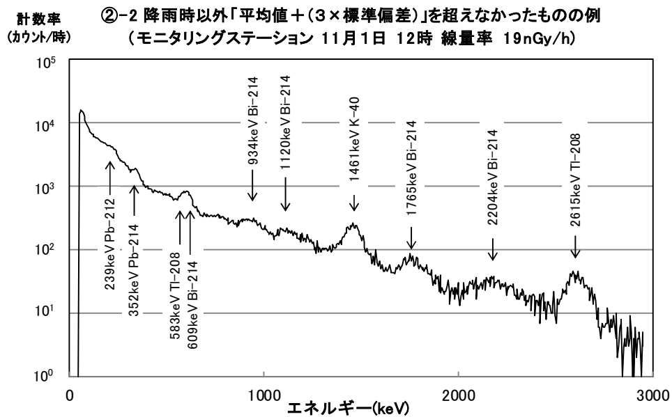
図 9-2 愛媛県測定局 (NaI (Tl) シンチレーション検出器) における 空間ガンマ線スペクトル図 (降雨時以外の例)
