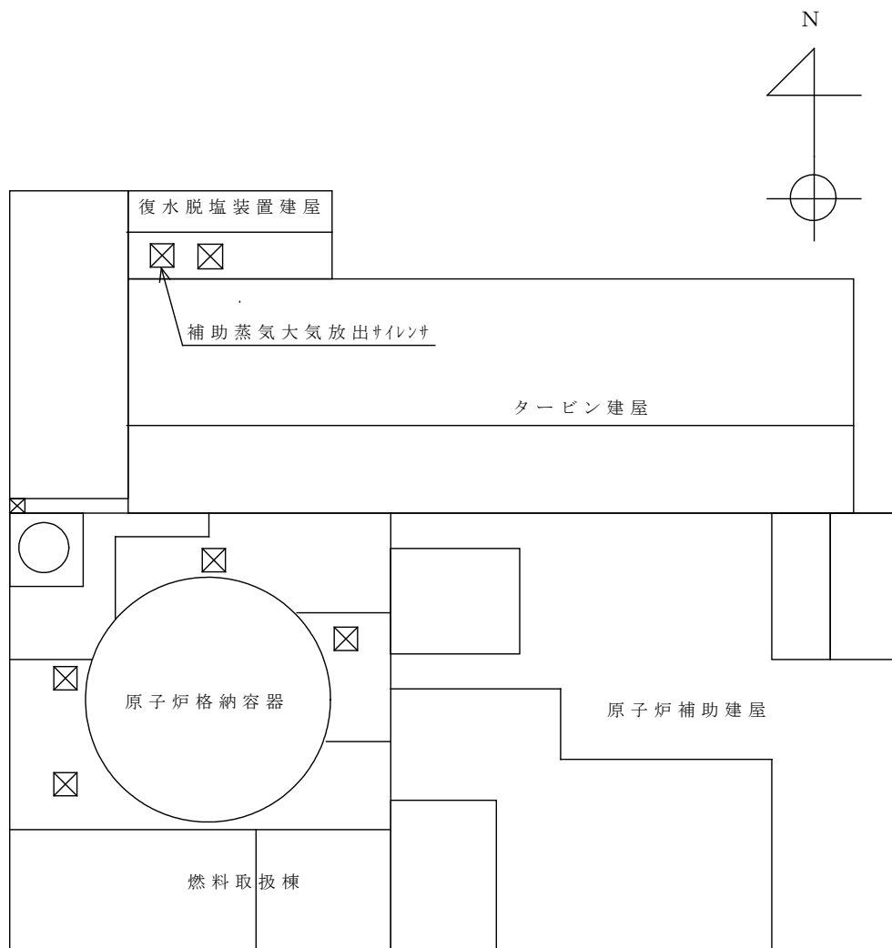
伊方発電所3号機 蒸気排気箇所配置図
