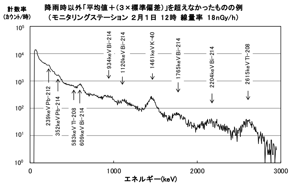
図 11 愛媛県測定局 (NaI(Tl)シンチレーション検出器) における 空間 \gamma 線スペクトル図 (降雨時以外の例)
