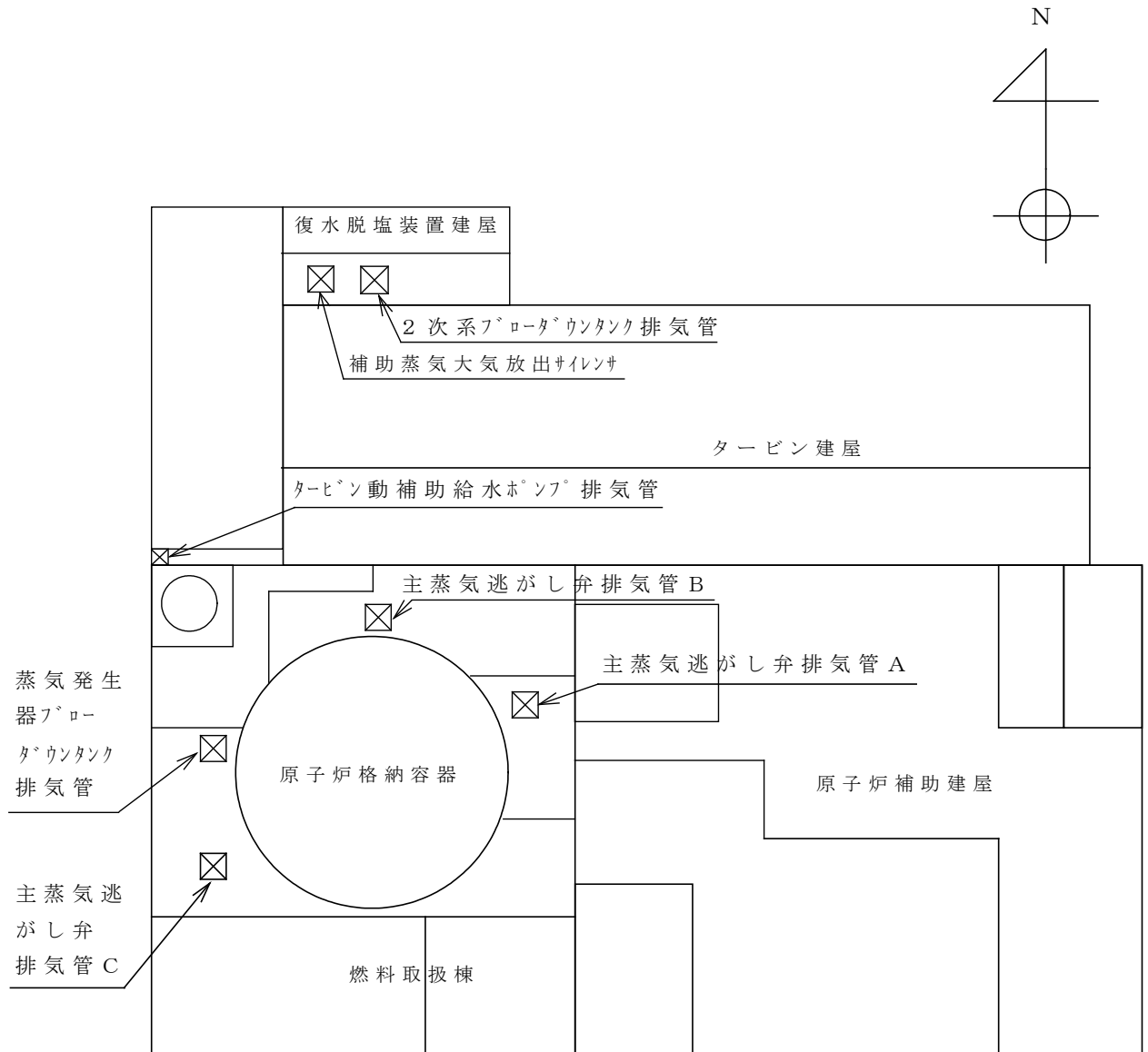
伊方発電所 3号機 蒸気排気箇所配置図
