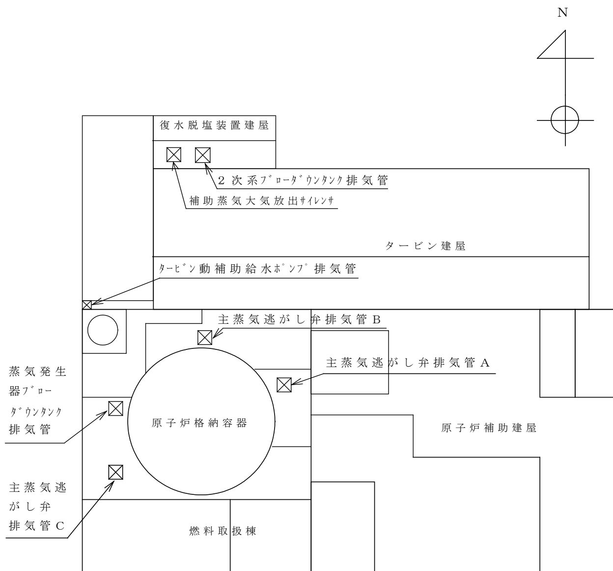
伊方発電所3号機 蒸気排気箇所配置図
