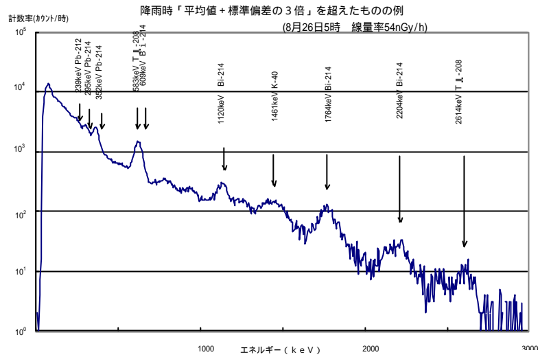
図14 愛媛県モニタリングステーションにおける空間ガンマ線スペクトル図(例)
