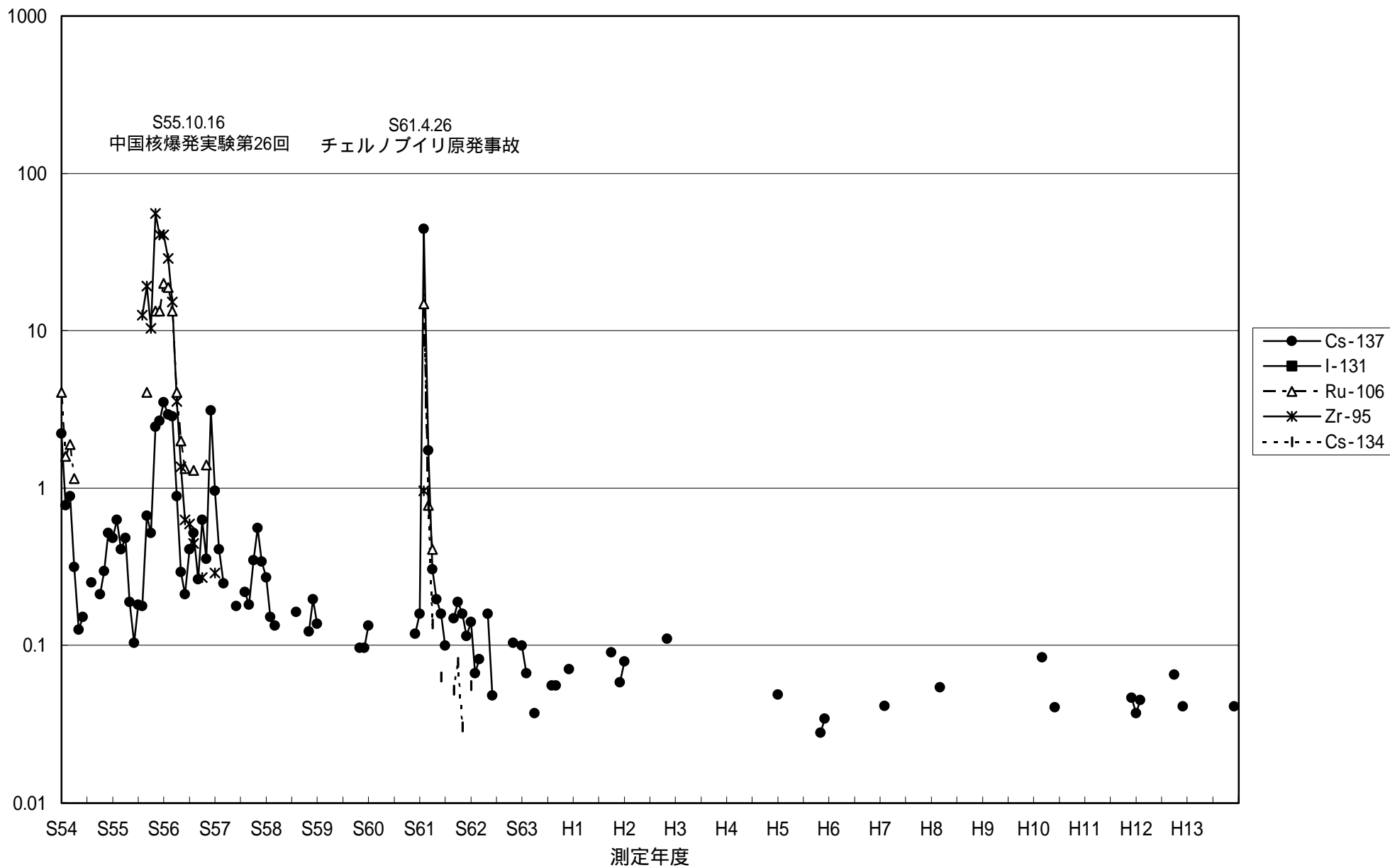
図31 降下物中の放射性核種の推移 [ 松山市 ( 愛媛県立衛生環境研究所 ) ]
