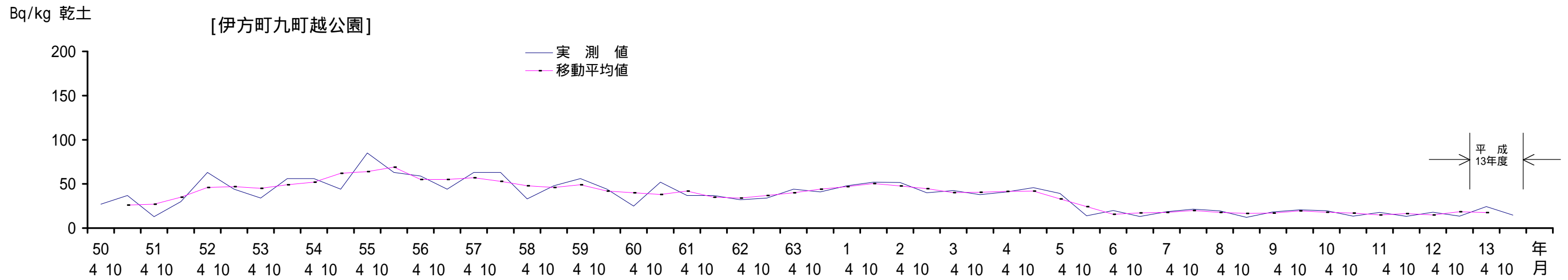
図35 土壌中のセシウム - 137の推移 (四国電力(株)測定分)
