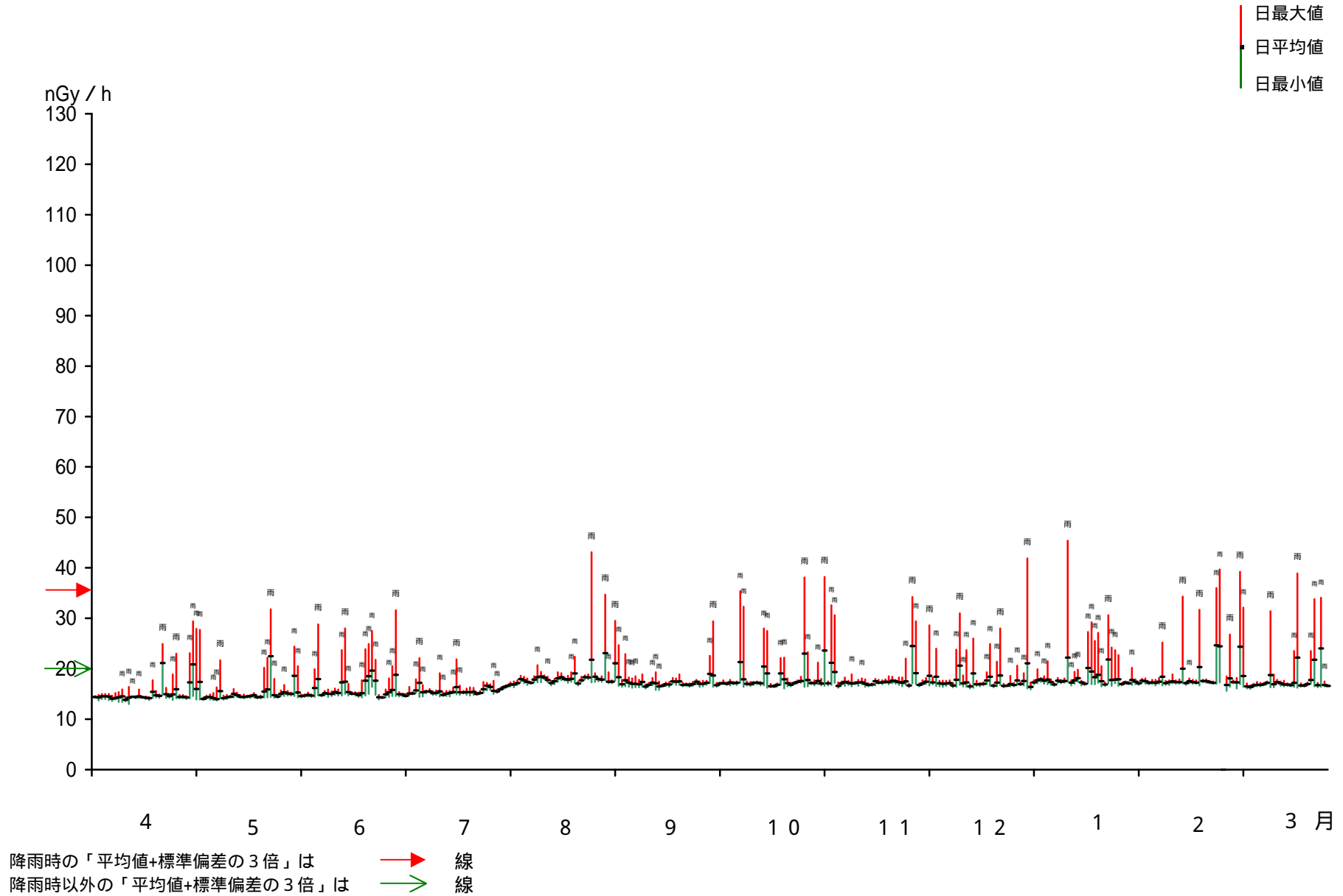
図21 愛媛県モニタリングポスト加周における空間線量率（1時間値）
