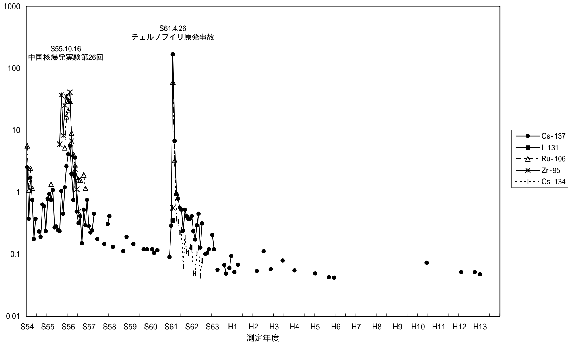
図30 降下物中の放射性核種の推移 [ 伊方町九町越公園 ]
