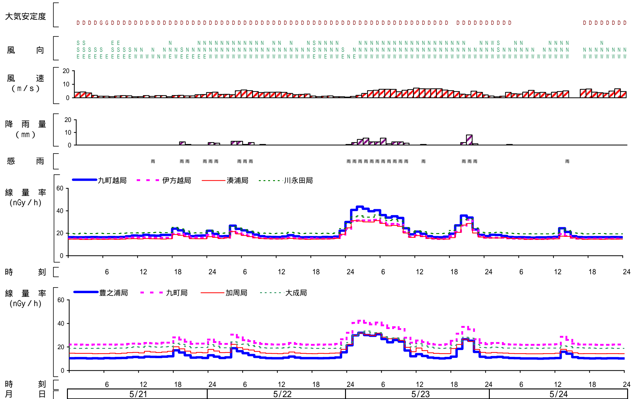
図6 降雨に対応して発生している線量率の変化例 平成13年5月21日～24日
