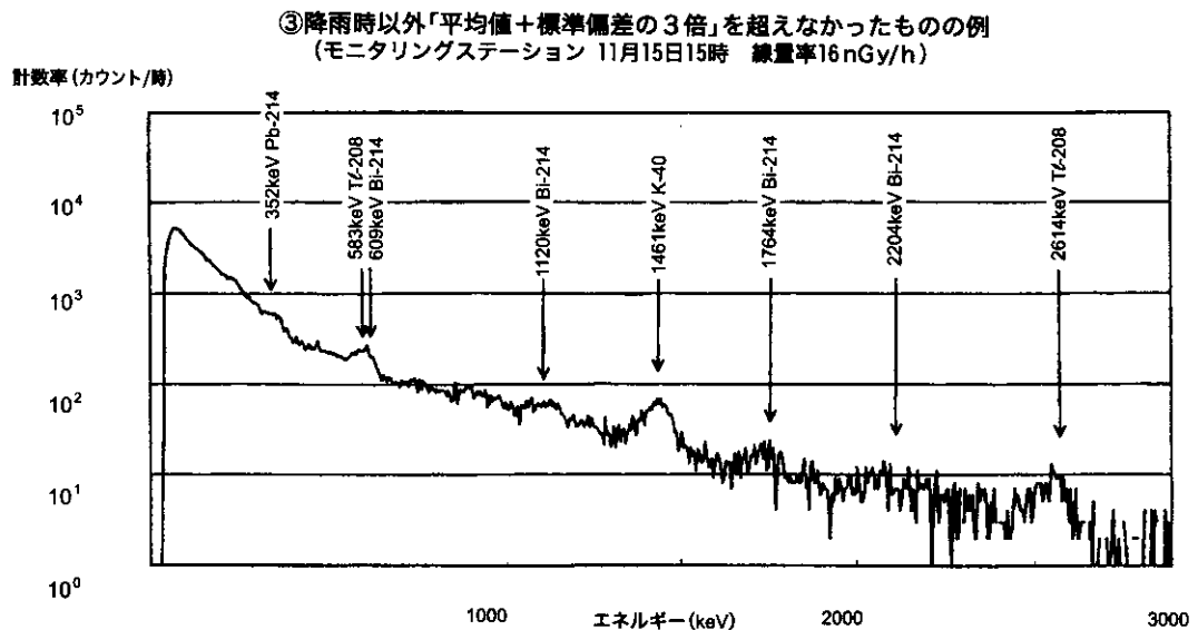
図7 愛媛県測定局における空間ガンマ線スペクトル図 (例)
