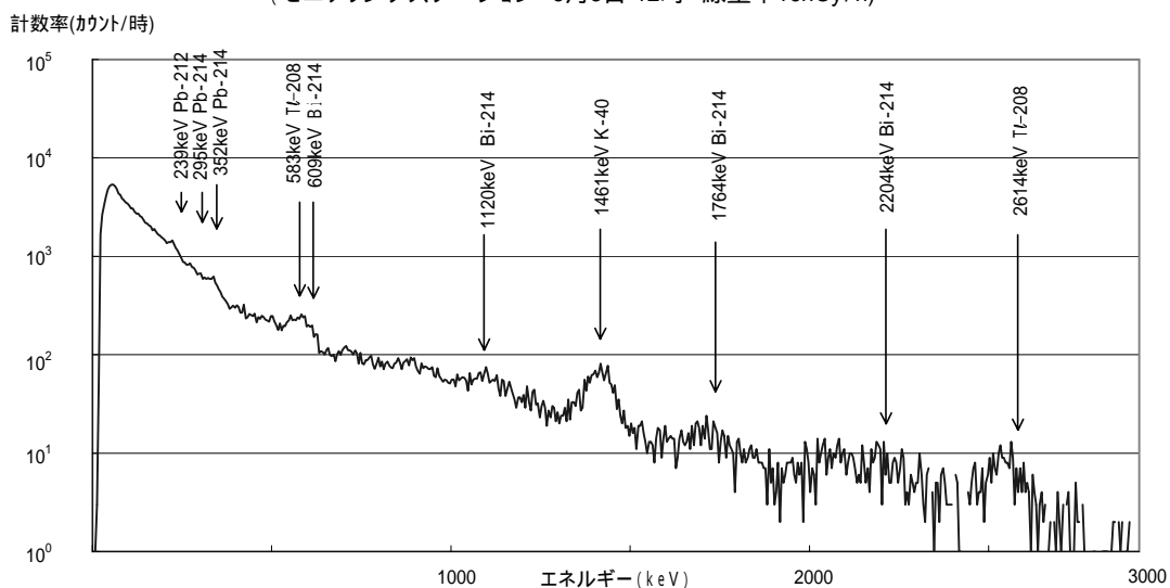
図7 愛媛県測定局における空間ガンマ線スペクトル図(例)
