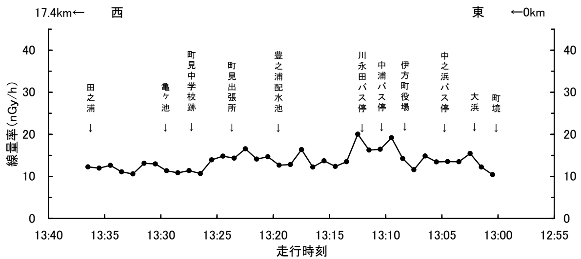
図1-2 モニタ車による空間線量率の走行測定
