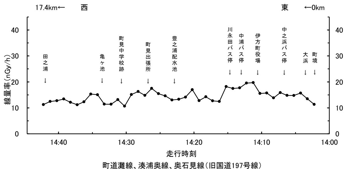
図1-2 モニタ車による空間線量率の走行測定(H24.5月実施分) (3"×3"NaI(Tl)シンチレーション検出器(エネルギー補償型))
