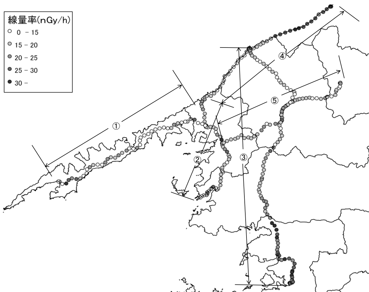
図1-1 3''\phi \times 3''\text{NaI} (T0) シンチレーション検出器 (エネルギー補償方式) による測定結果(地図上データ表示)
