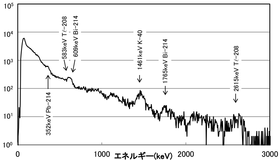
図8 愛媛県測定局における空間ガンマ線スペクトル図(例)
