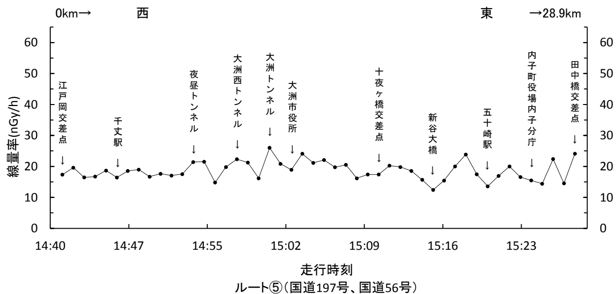
図1-2 3''\phi \times 3''\text{NaI (Tl)} シンチレーション検出器 (エネルギー補償方式) による測定結果 (時系列グラフ)
