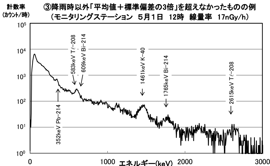
図8 愛媛県測定局における空間ガンマ線スペクトル図(例)
