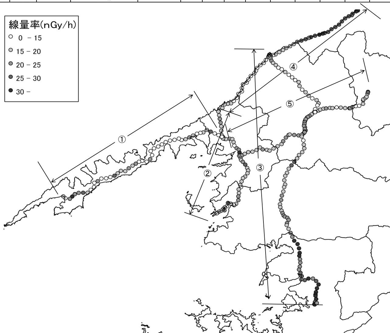
図1-1 3"φ×3"Nal(Tl)シンチレーション検出器(エネルギー補償方式)による 測定結果(地図上データ表示)
