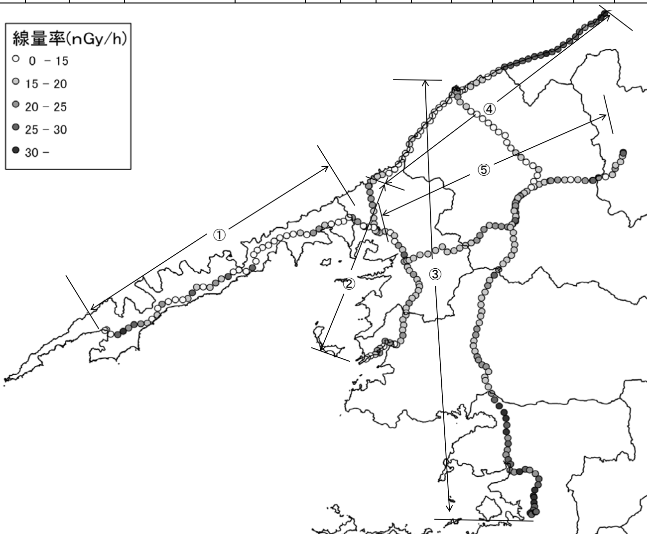
図2-1 3"φ×3"Nal(Tl)シンチレーション検出器(エネルギー補償方式)による測定結果(地図上データ表示)
