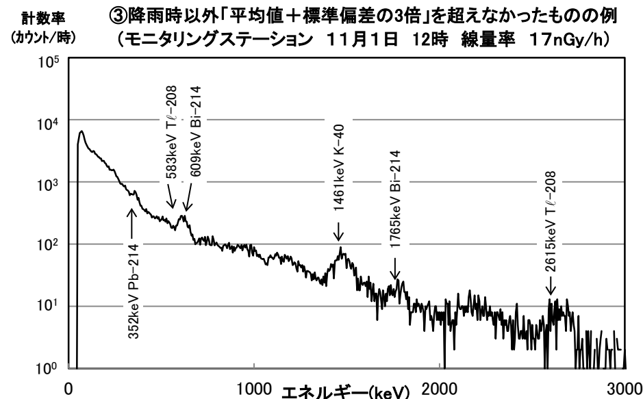
図9 愛媛県測定局における空間ガンマ線スペクトル図(例)
