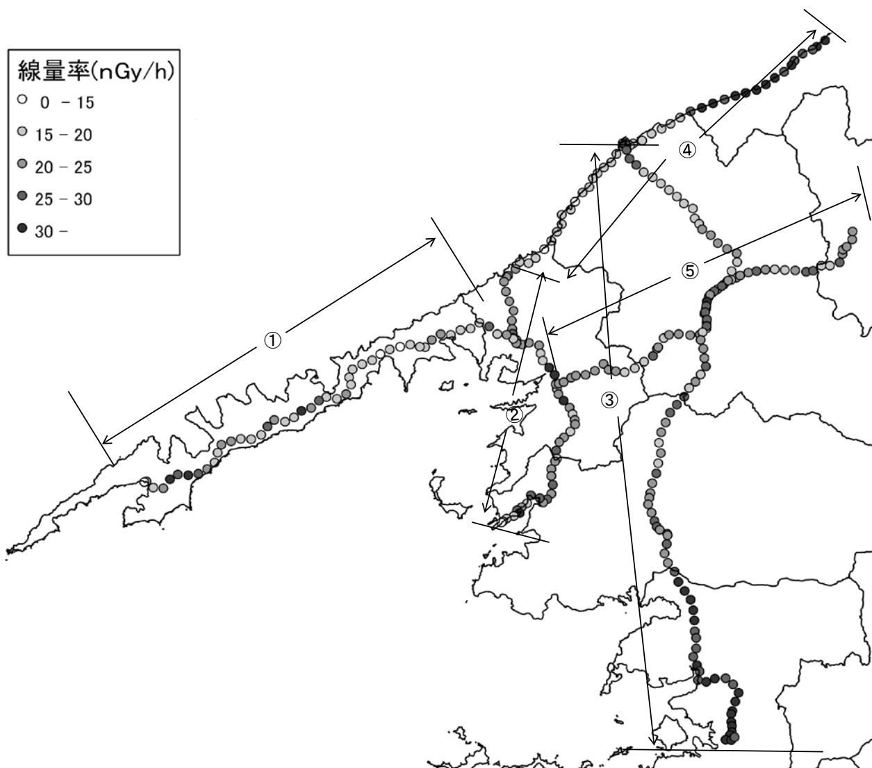
図2-1 3"φ×3"NaI(Tl)シンチレーション検出器(エネルギー補償型)による測定結果(地図上データ表示)
