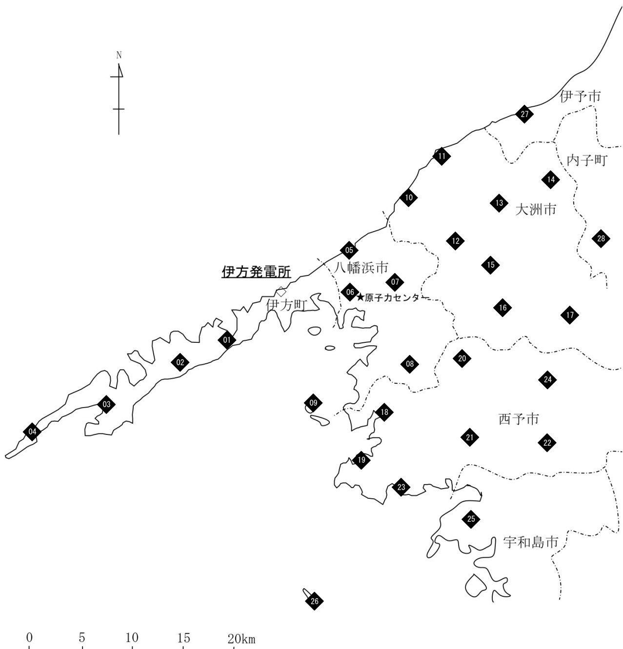
図9 土壌 調査地点図
