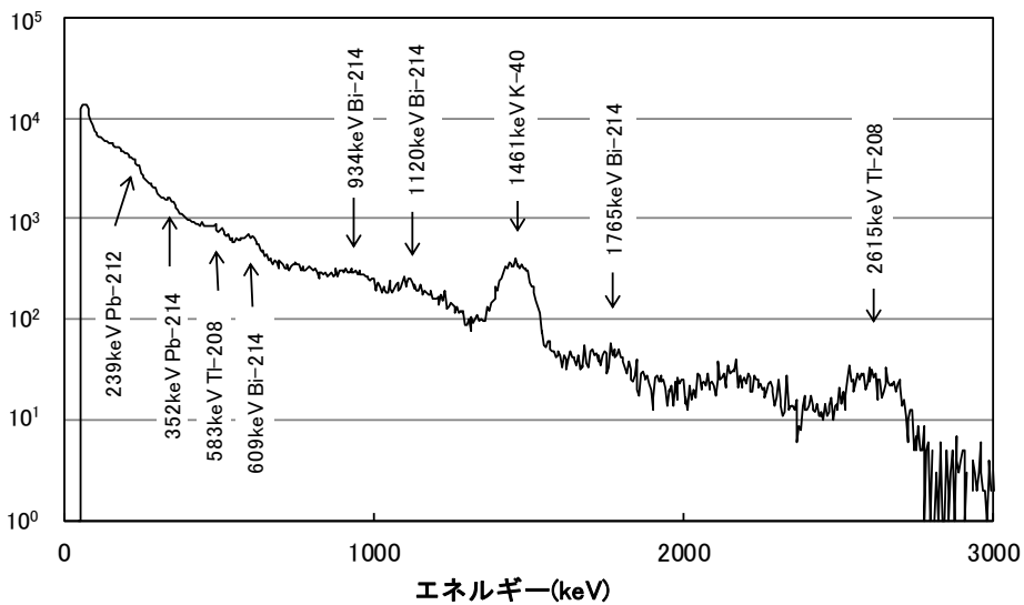
①-2 降雨時以外「平均値+(3×標準偏差)」を超えなかったものの例 (伊方越局 8月1日 12時 線量率 18nGy/h)
