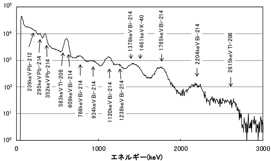
①-1 降雨時「平均値+(3×標準偏差)」を超えたものの例 (伊方越局 7月6日 8時 線量率 72nGy/h)
