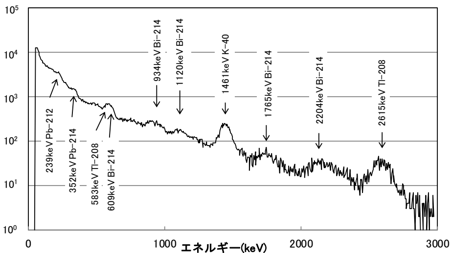
図9-2 愛媛県測定局における空間ガンマ線スペクトル図 (降雨時以外の例)
