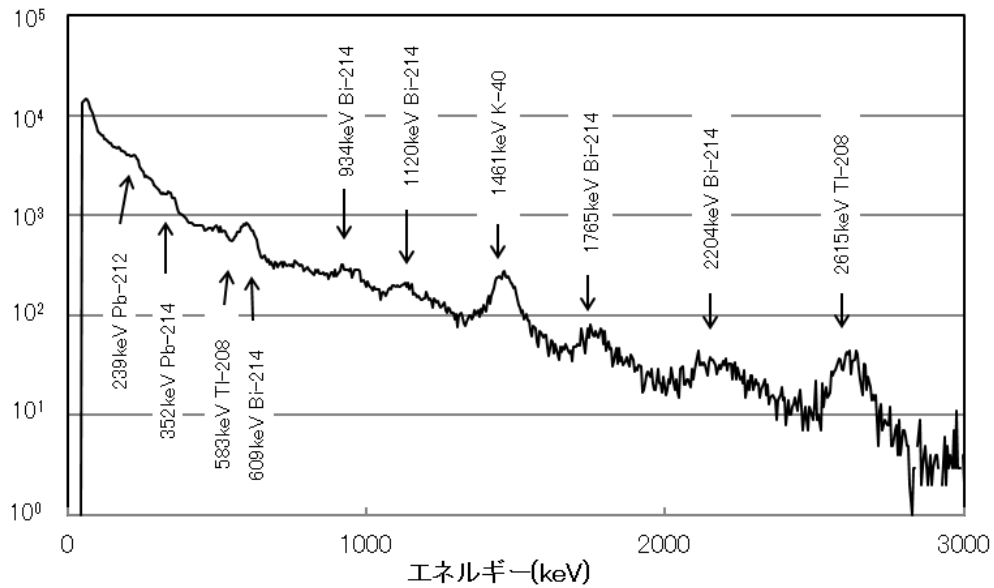
図9-2 愛媛県測定局における空間ガンマ線スペクトル図（降雨時以外の例）
