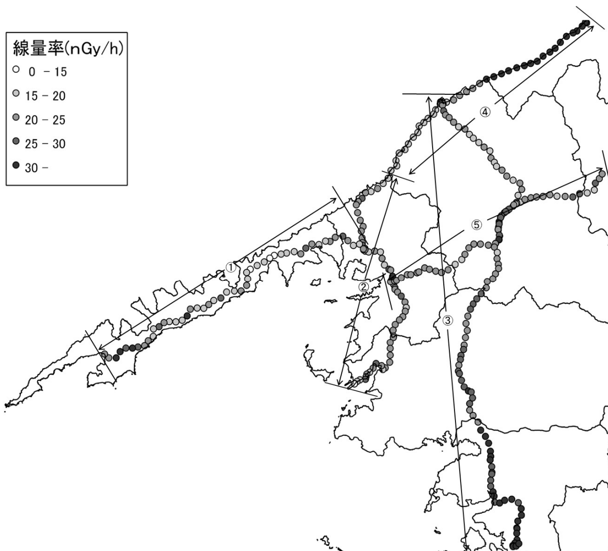
図2-1 3"φ×3"NaI（Tl）シンチレーション検出器（エネルギー補償方式）による測定結果 （地図上データ表示）
