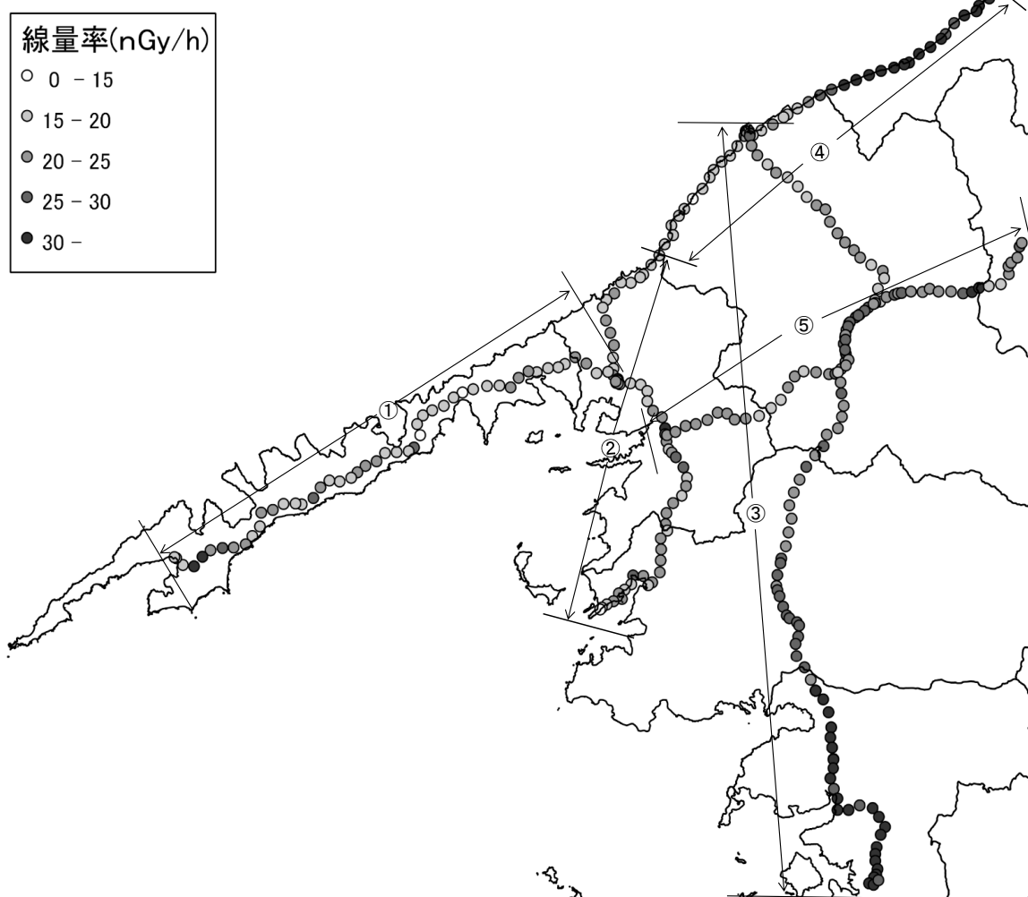
図2-1 3"φ×3"N a I（Tl）シンチレーション検出器による測定結果（地図上データ表示）
