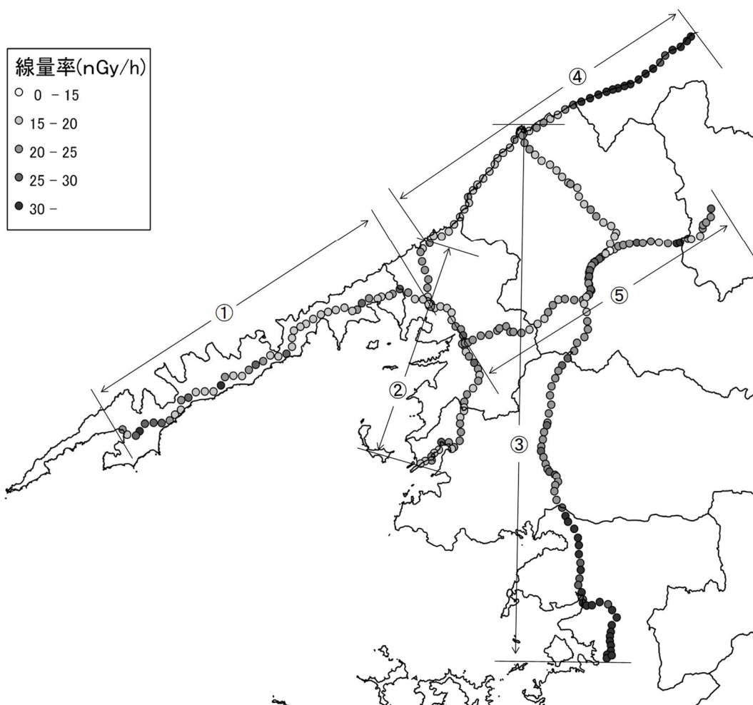
図2-1 3"φ×3"NaI (Tl) シンチレーション検出器 (温度補償・エネルギー補償回路付) による測定結果 (地図上データ表示)
