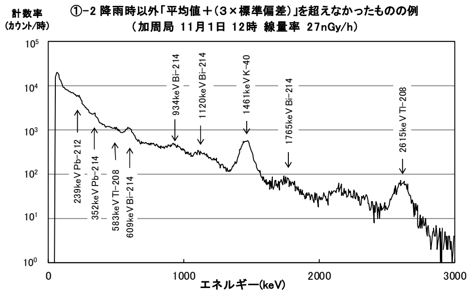
図 9-1 愛媛県測定局 (NaI (Tl) シンチレーション検出器) における 空間ガンマ線スペクトル図 (降雨時の例)
