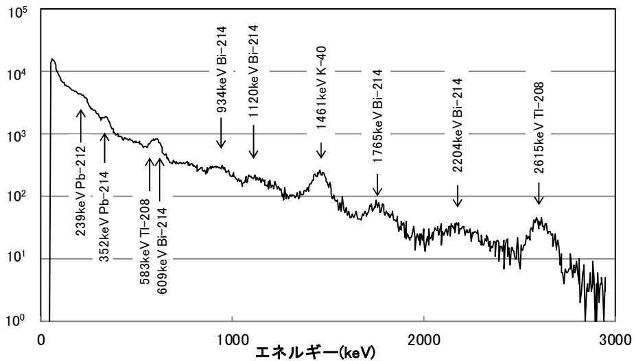
図 9-2 愛媛県測定局 (NaI (Tl) シンチレーション検出器) における 空間ガンマ線スペクトル図 (降雨時以外の例)
