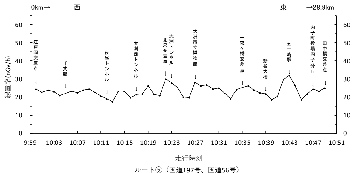
図2-2 3"φ×3"NaI (Tl) シンチレーション検出器（温度補償・エネルギー補償回路付）による測定結果（時系列グラフ）（令和4年3月測定結果）
