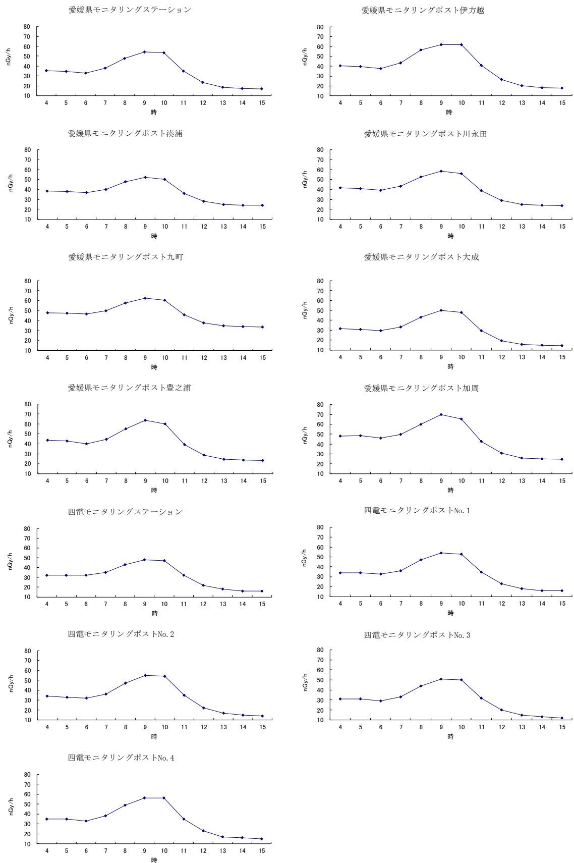
図 12 異なる方位のモニタに同時に発生している例（1 時間平均値） (NaI(Tl)シンチレーション検出器)（令和 3 年 5 月 27 日）
