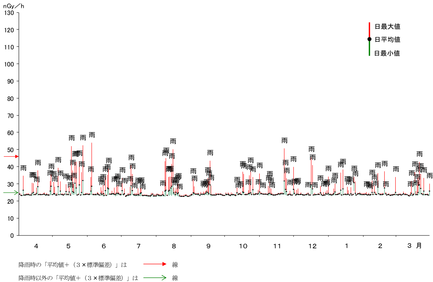
図 18 愛媛県モニタリングポスト湊浦における線量率（1 時間平均値）
