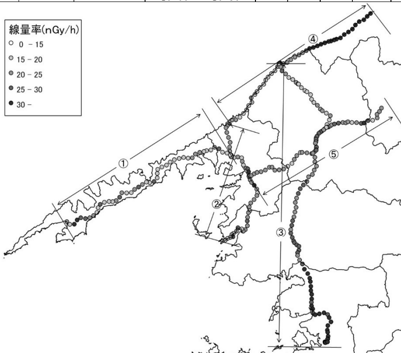
図2-1 3"φ×3"NaI(Tl)シンチレーション検出器（温度補償・エネルギー補償回路付）による測定結果（地図上データ表示）（令和4年3月測定結果）
