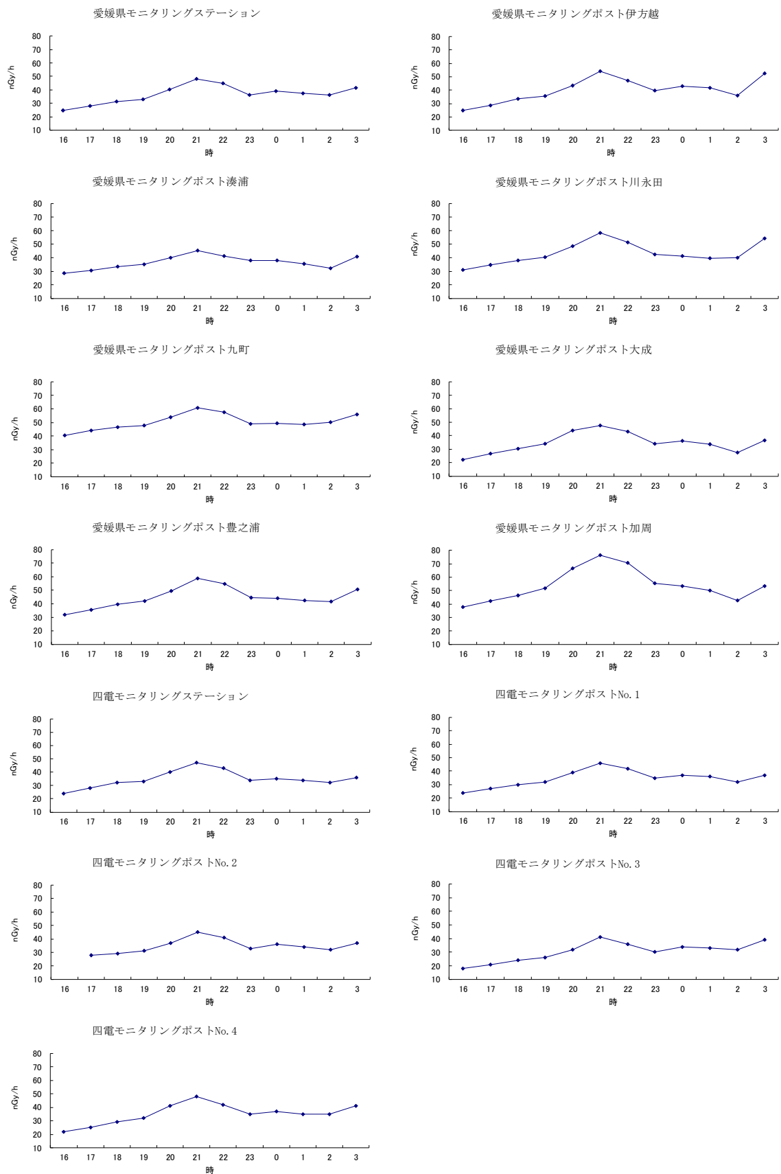
図 14 異なる方位のモニタに同時に発生している例（1 時間平均値） (NaI(Tl)シンチレーション検出器)（令和 3 年 12 月 16 日～令和 3 年 12 月 17 日）
