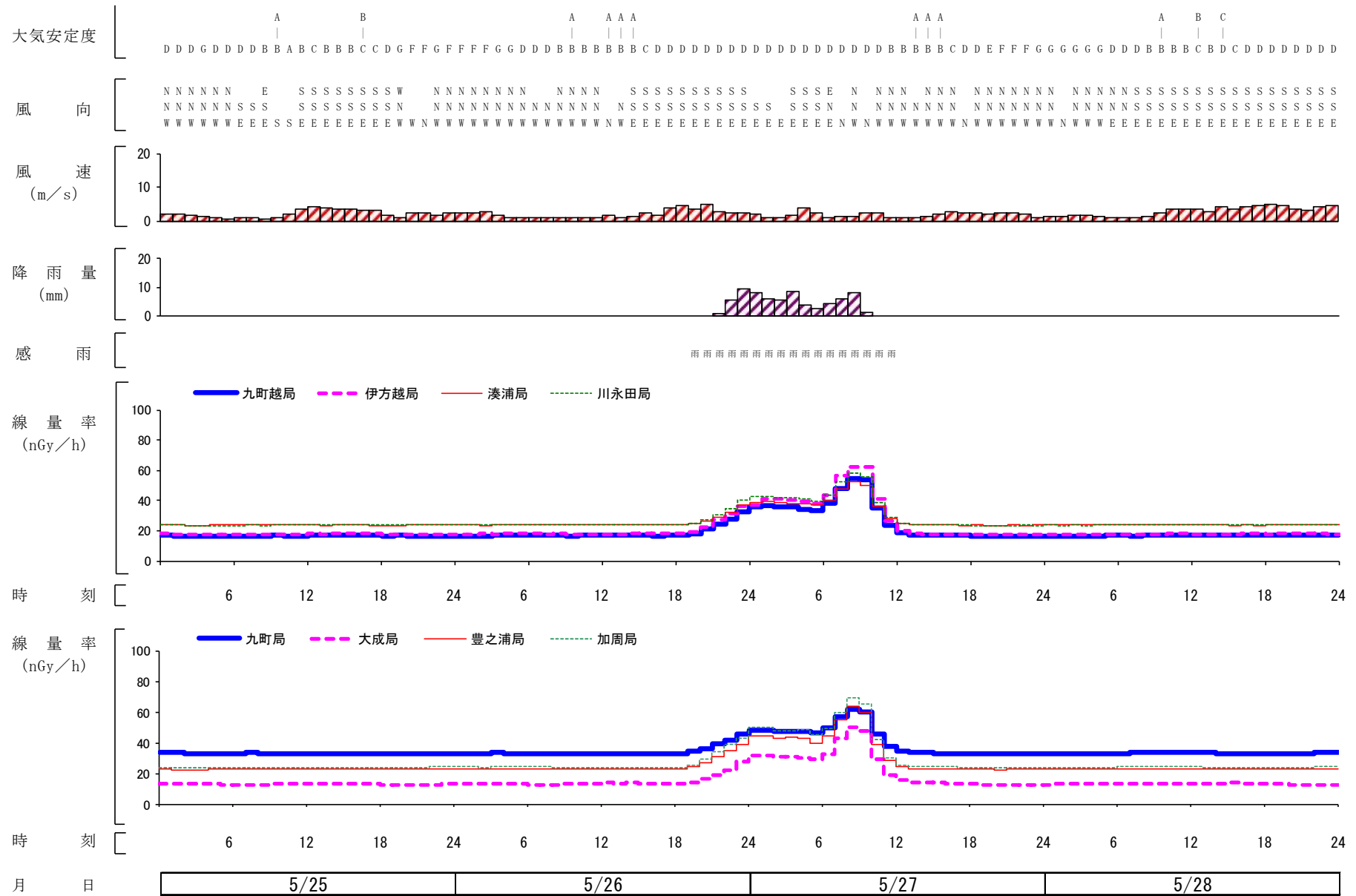
図9 降雨に対応して発生している線量率（1時間平均値）の変化例（令和3年5月25日～令和3年5月28日）
