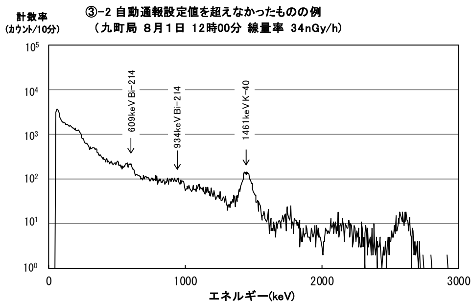
図 31 愛媛県測定局 (NaI(Tl)シンチレーション検出器) における 空間ガンマ線スペクトル図 (自動通報設定値超過時の例)
