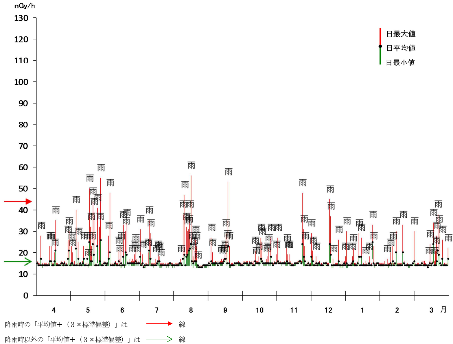
図 26 四国電力モニタリングポスト No.2 における線量率（1 時間平均値）
