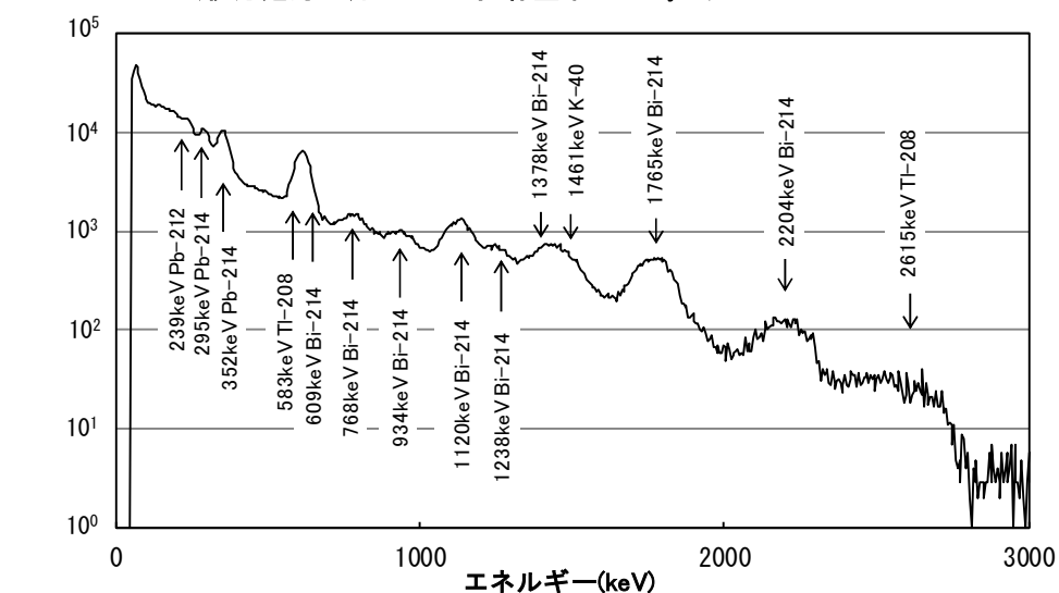
①-1 降雨時「平均値＋(3×標準偏差)」を超えたものの例 (伊方越局 8月15日 5時 線量率 73nGy/h)
