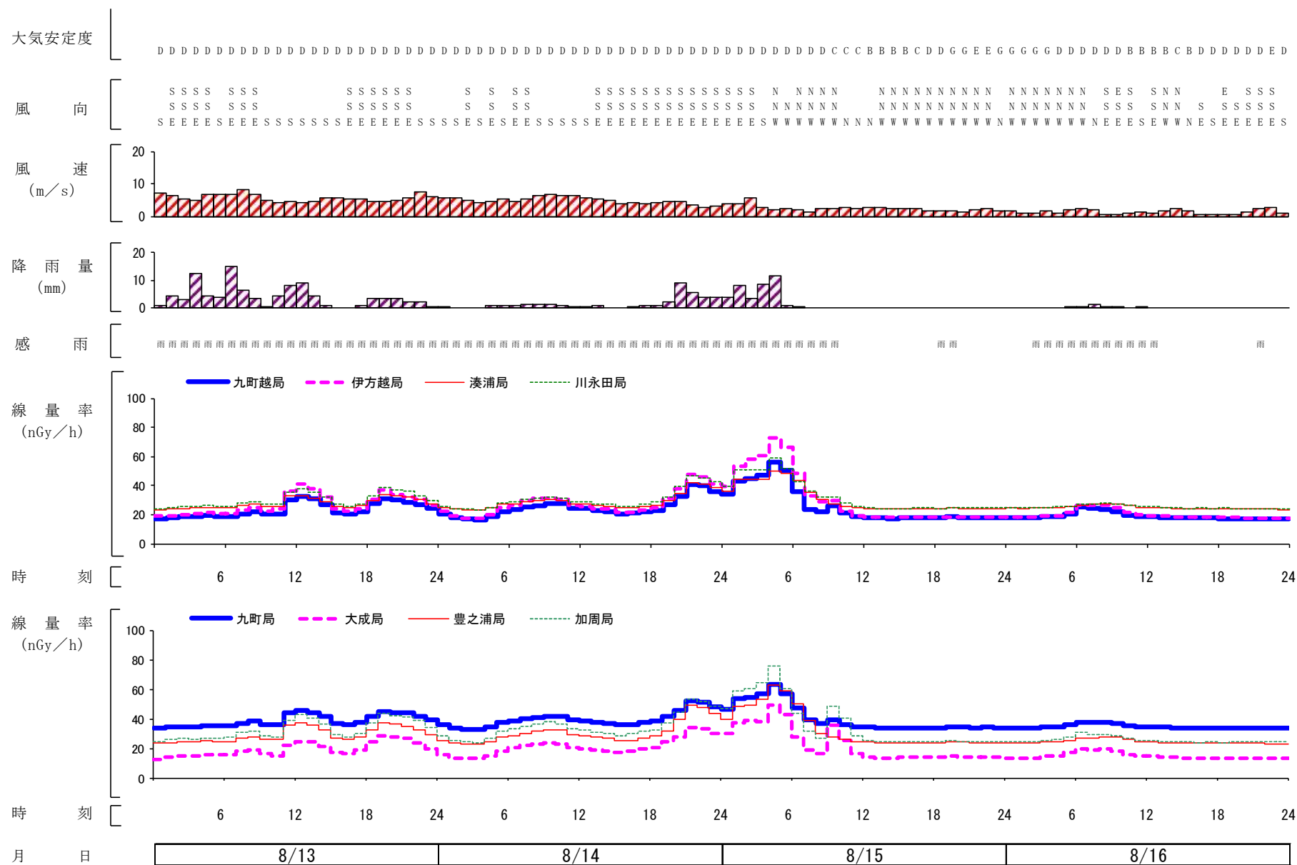
図 10 降雨に対応して発生している線量率（1時間平均値）の変化例（令和3年8月13日～令和3年8月16日）
