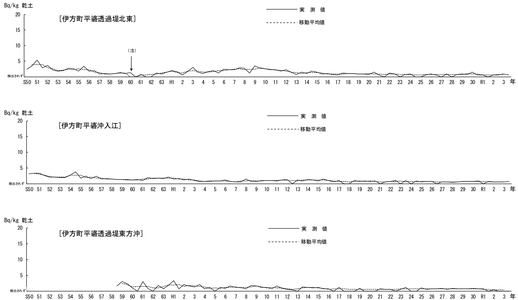
図 38 海底土中のセシウム-137 濃度の推移（四国電力株測定分）
