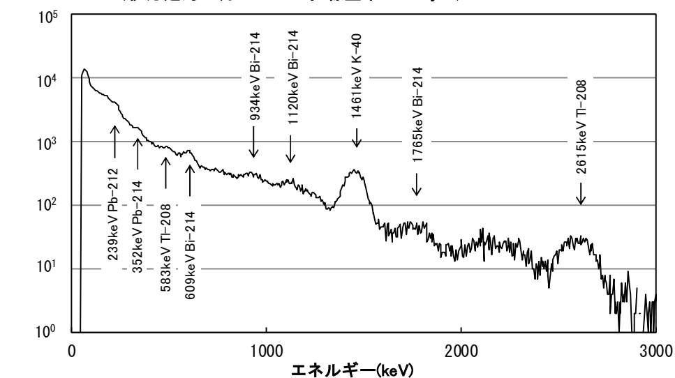
①-2 降雨時以外「平均値＋(3×標準偏差)」を超えなかったものの例 (伊方越局 8月1日 12時 線量率 19nGy/h)
