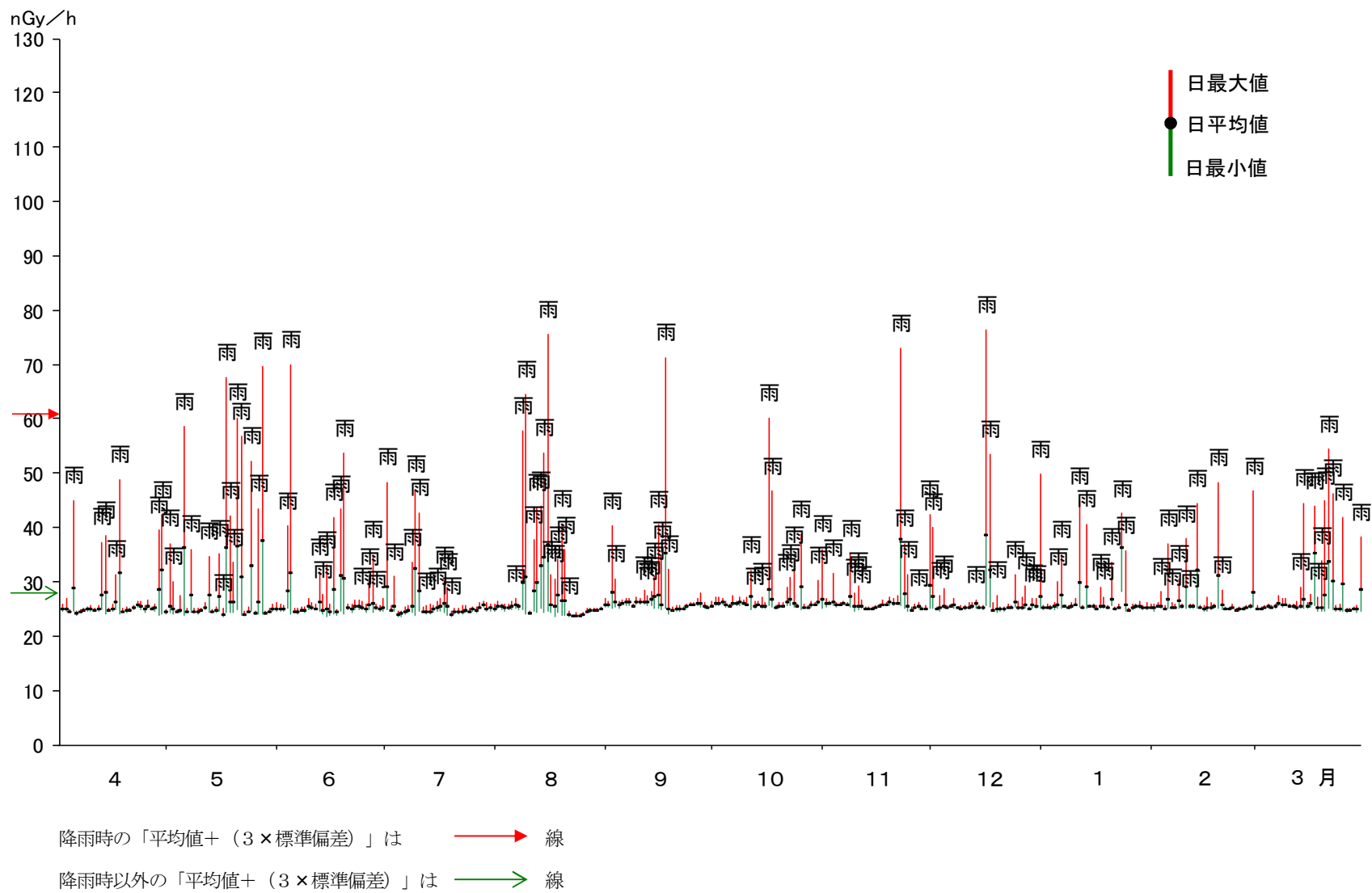
図 23 愛媛県モニタリングポスト加周における線量率（1 時間平均値）
