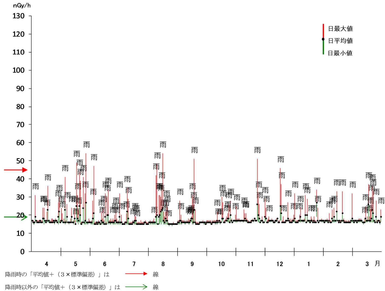
図 25 四国電力モニタリングポスト No.1 における線量率（1 時間平均値）
