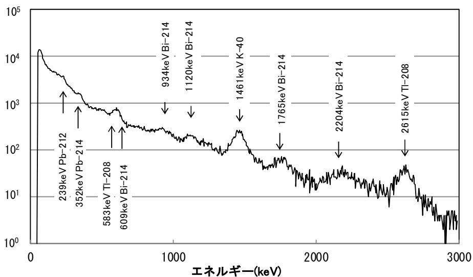
計数率 (カウント/時) ②-2 降雨時以外「平均値＋標準偏差の3倍」を超えなかったものの例 (モニタリングステーション 5月1日 12時 線量率 17nGy/h)
