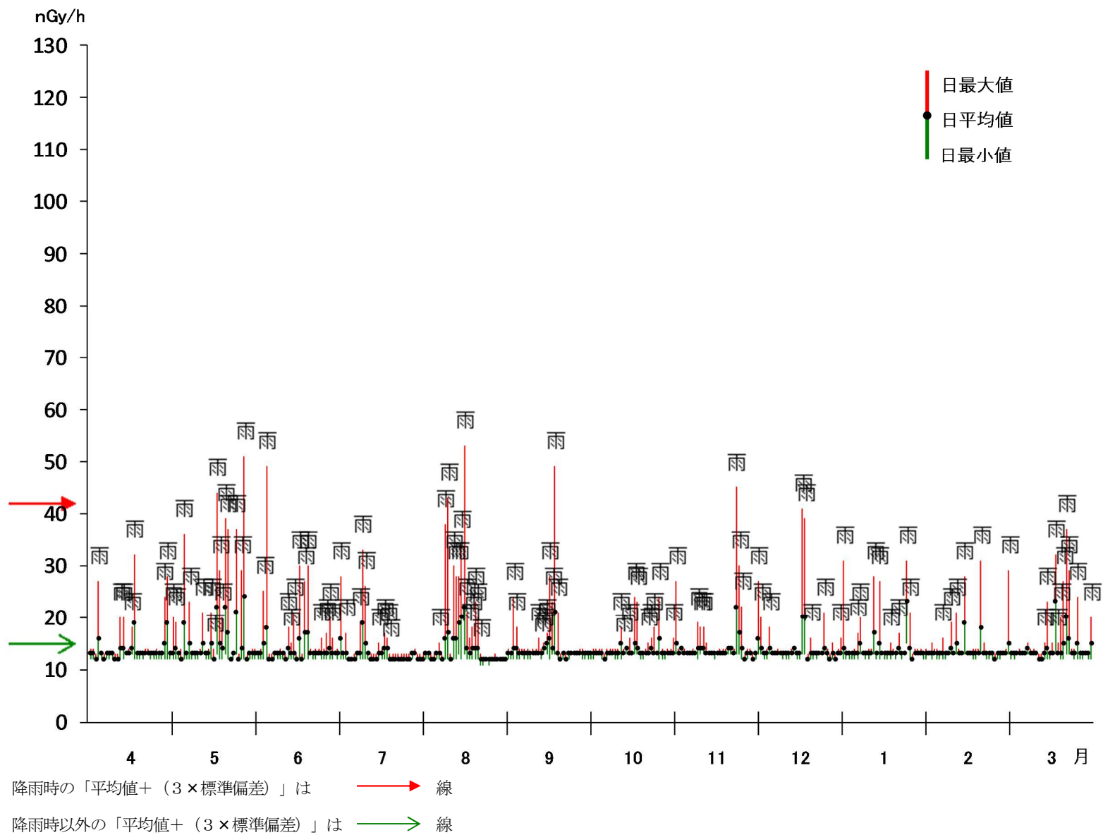
図 27 四国電力モニタリングポスト No.3 における線量率（1 時間平均値）
