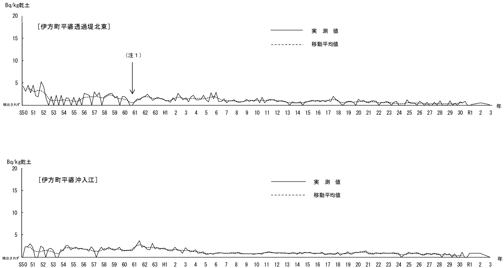
図 36 海底土中のセシウム-137 濃度の推移（愛媛県測定分）
