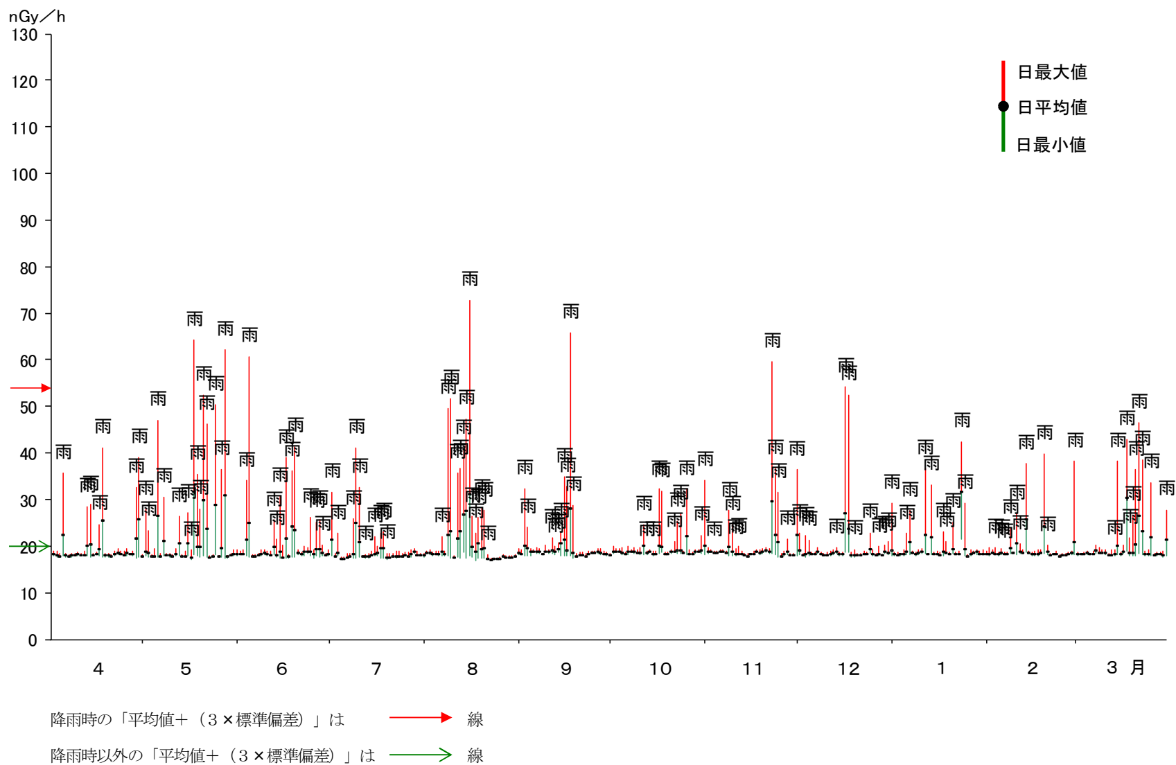
図 17 愛媛県モニタリングポスト伊方越における線量率（1 時間平均値）
