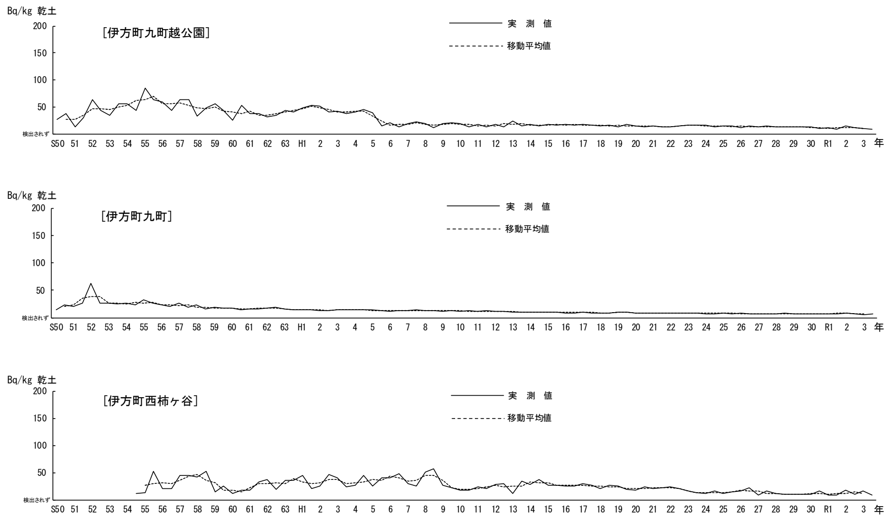
図 37 土壤中のセシウム-137 濃度の推移 (四国電力株測定分)
