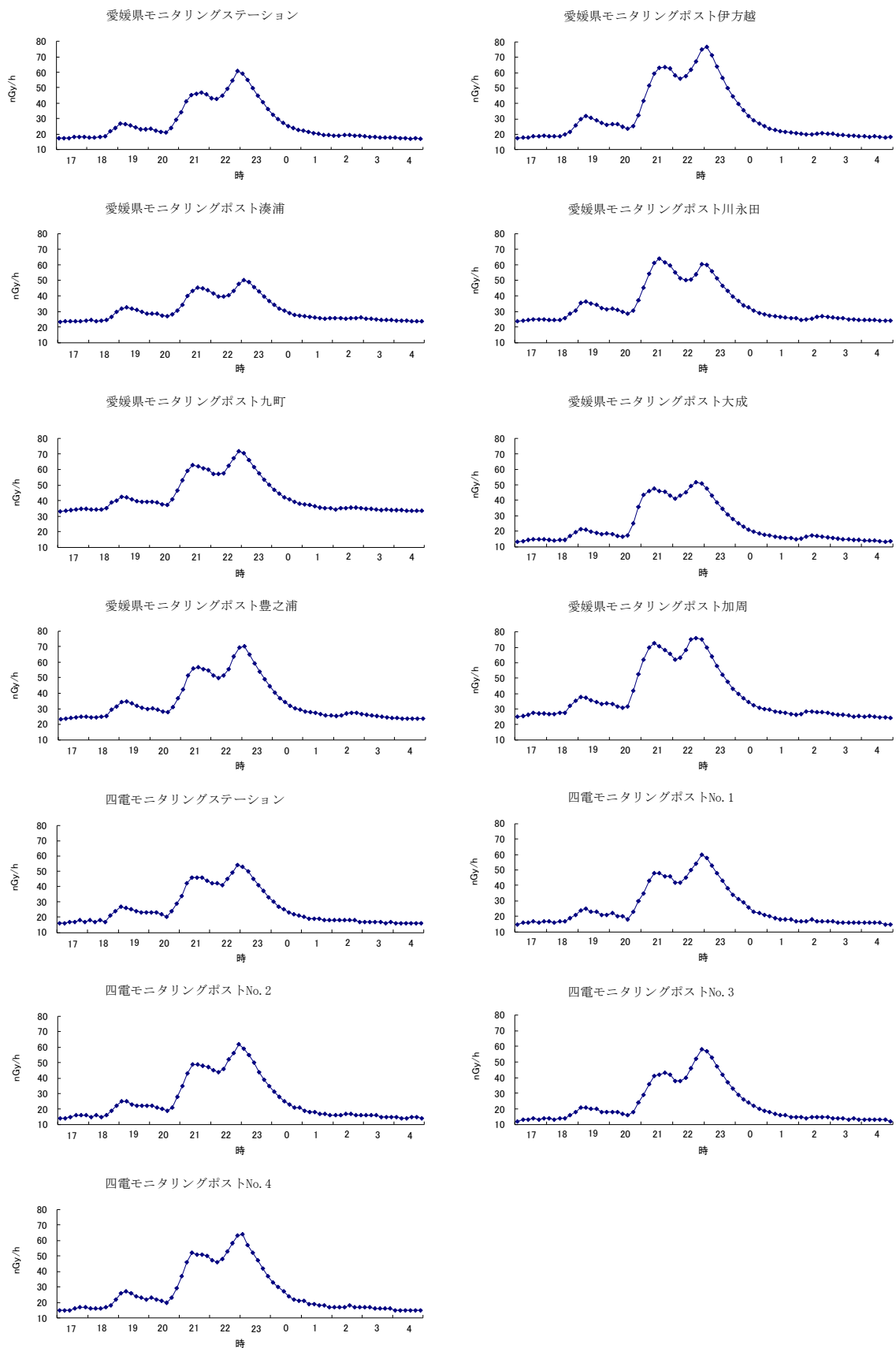
図 30 異なる方位のモニタに同時に発生している例（10 分間平均値） （NaI(Tl)シンチレーション検出器）（令和 3 年 9 月 17 日～令和 3 年 9 月 18 日）
