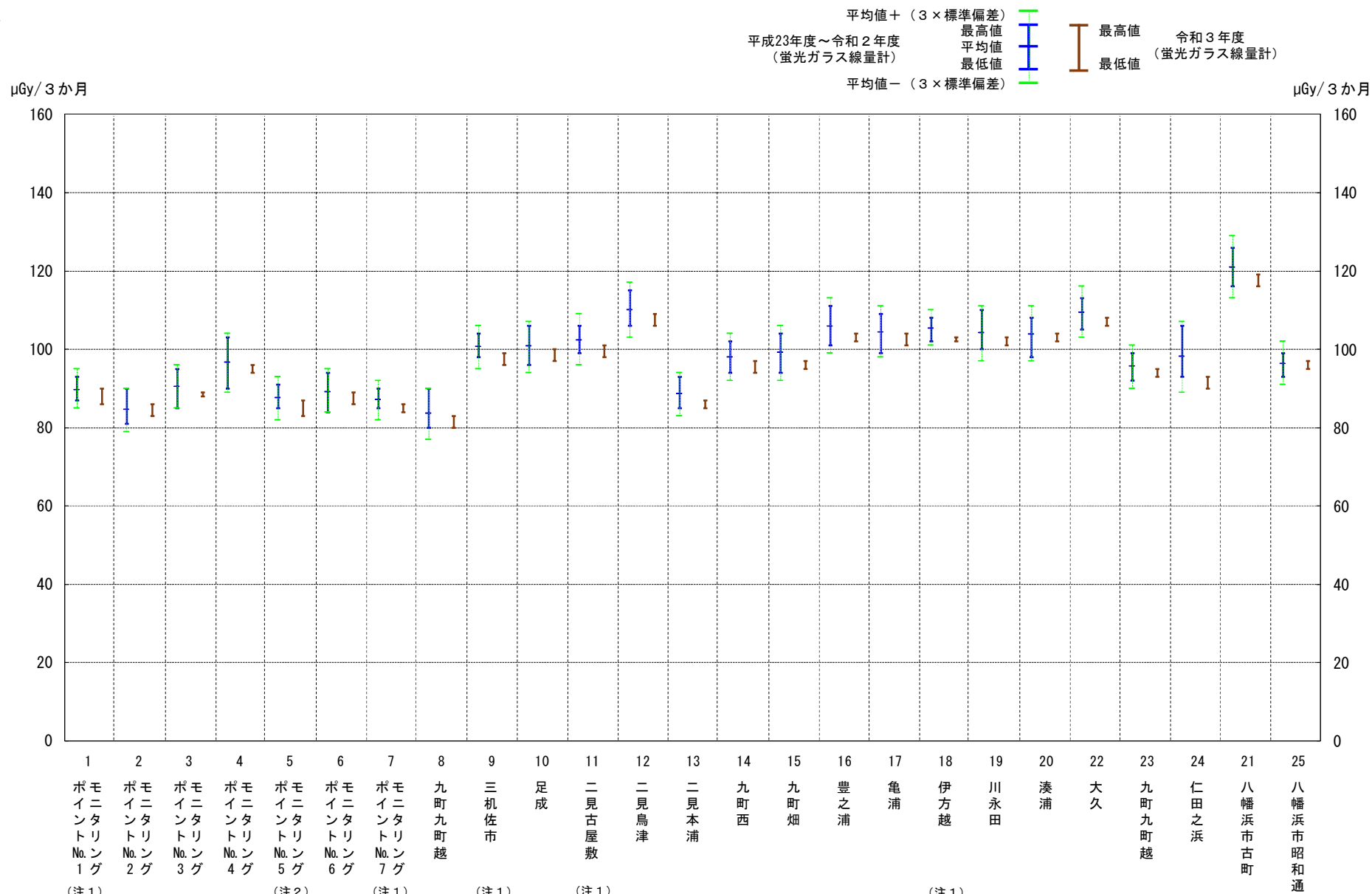
図 33 積算線量測定結果の過去における測定値との比較図（四国電力㈱測定分）
