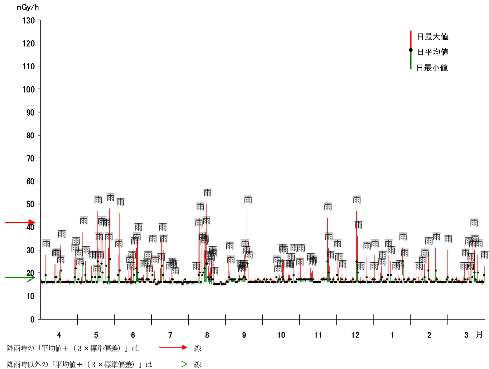
図 24 四国電力モニタリングステーションにおける線量率（1 時間平均値）
