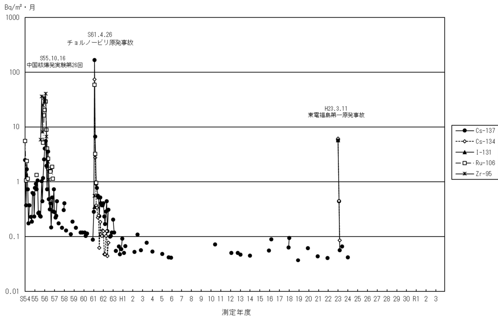
図 34 降下物中の放射性核種濃度の推移 [伊方町九町越公園]
