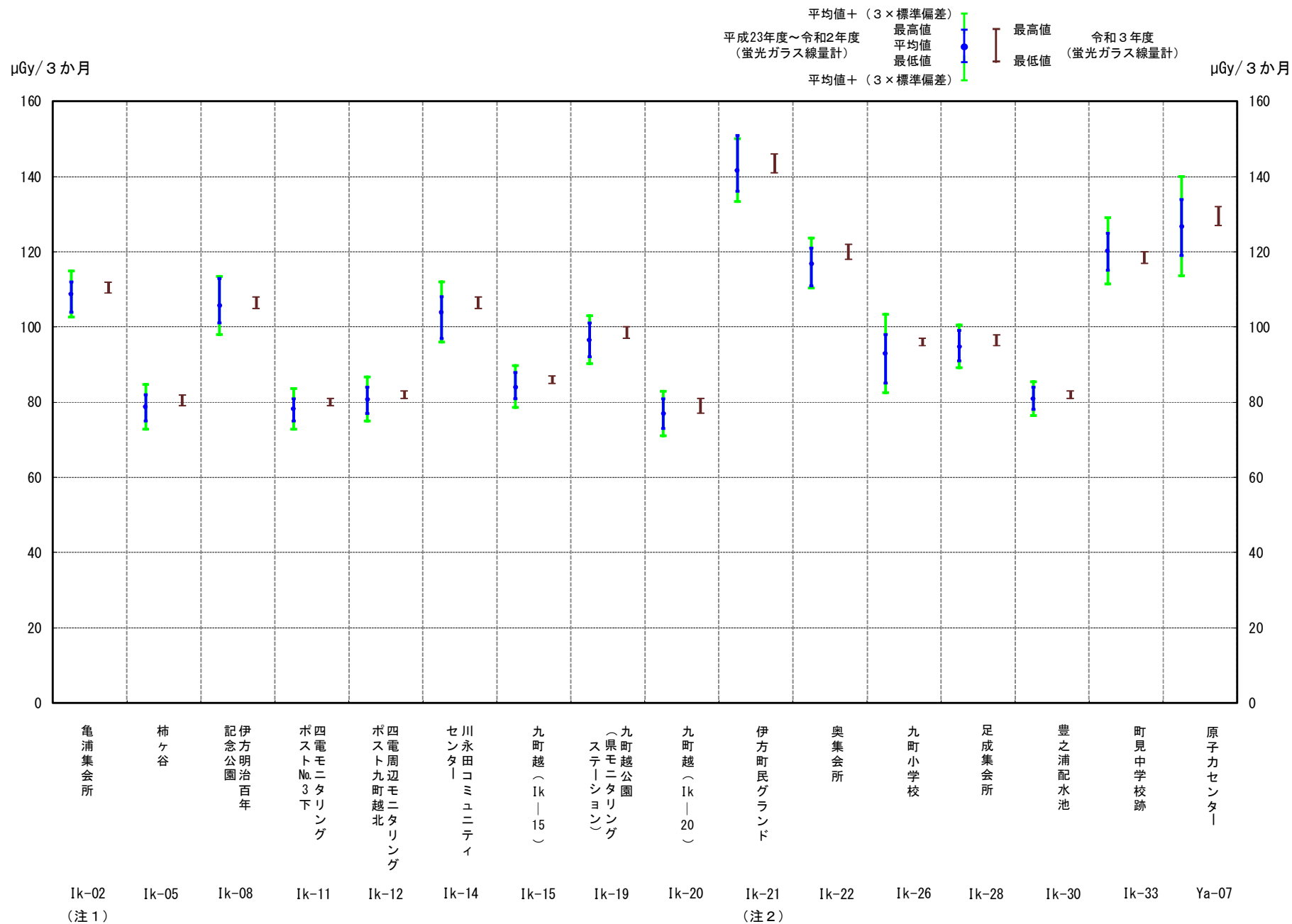
図 32 積算線量測定結果の過去における測定値との比較図 (愛媛県測定分)
