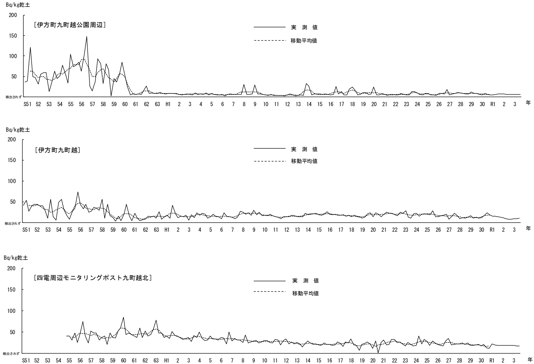
図 35 土壤中のセシウム-137 濃度の推移（愛媛県測定分）
