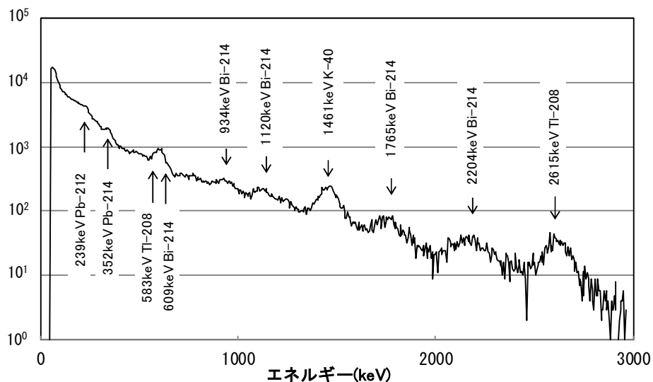
計数率 (カウント/時) ②-1 降雨時以外「平均値＋標準偏差の3倍」を超えたものの例 (モニタリングステーション 6月22日 10時 線量率 20nGy/h)
