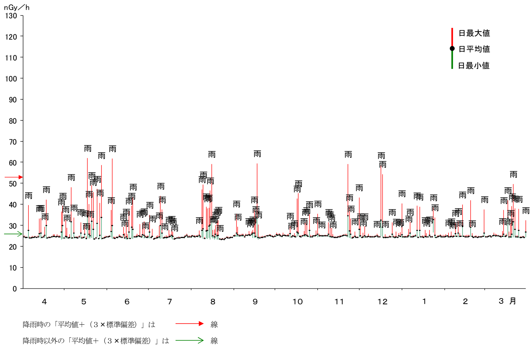
図 19 愛媛県モニタリングポスト川永田における線量率（1 時間平均値）
