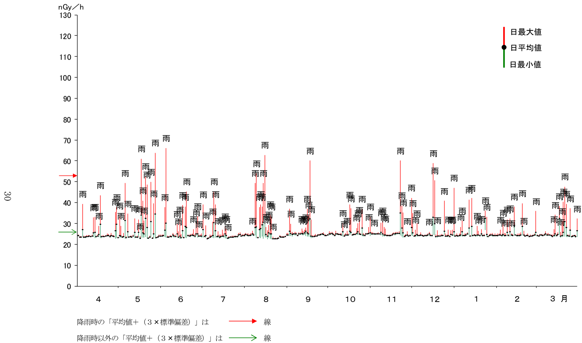
図 22 愛媛県モニタリングポスト豊之浦における線量率（1 時間平均値）
