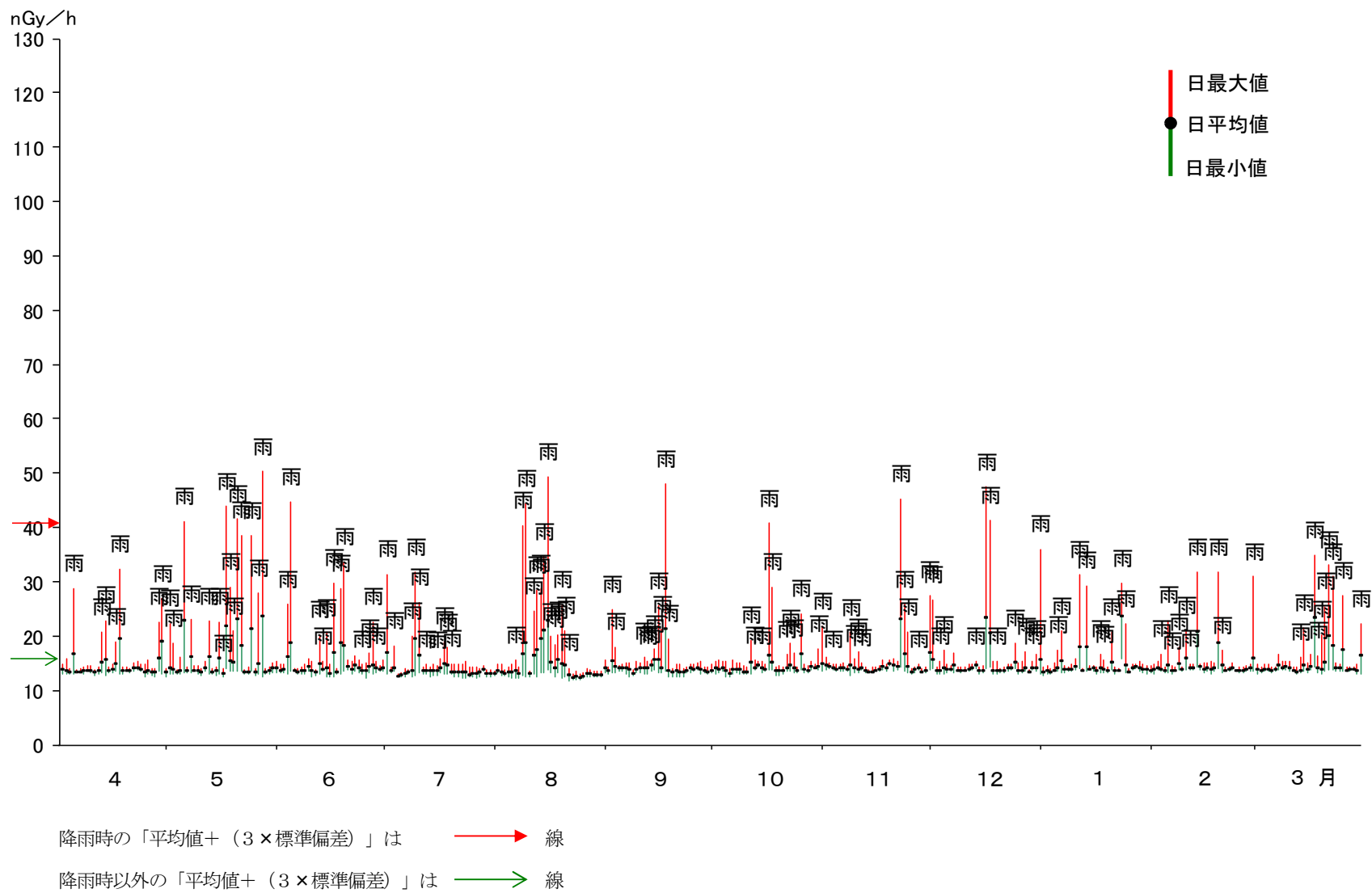
図 21 愛媛県モニタリングポスト大成における線量率（1 時間平均値）
