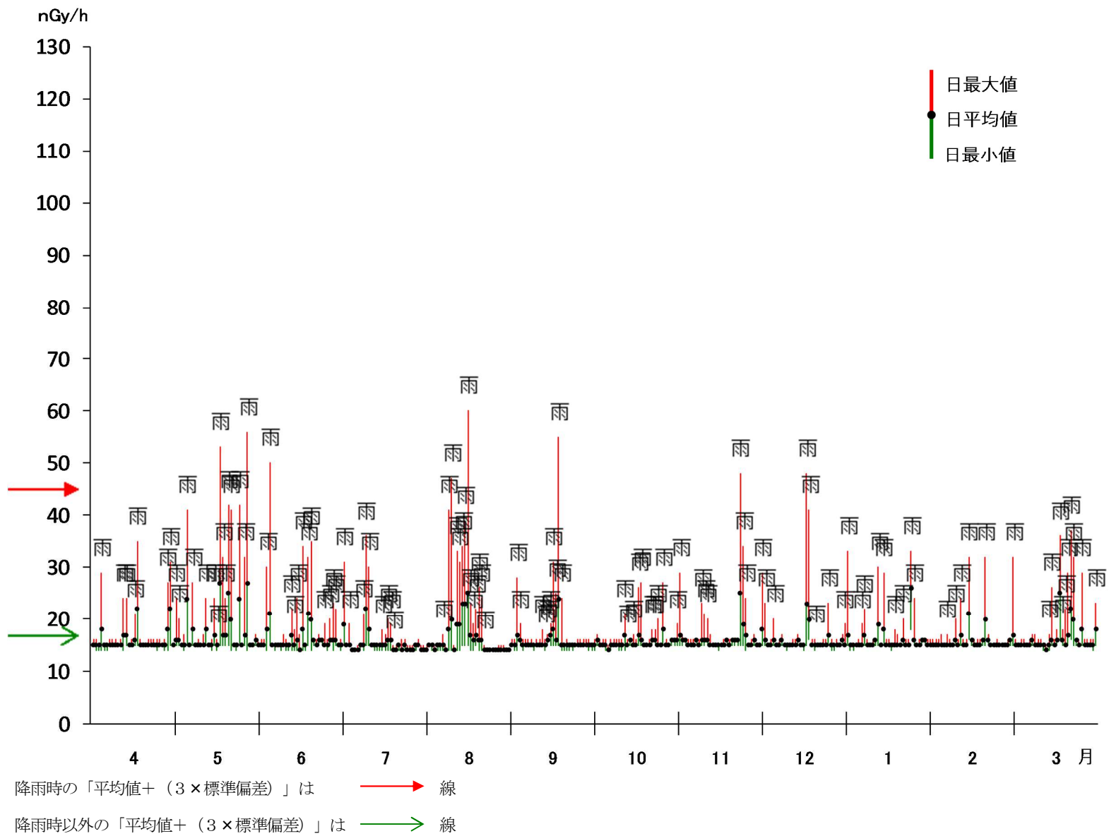
図 28 四国電力モニタリングポスト No.4 における線量率（1 時間平均値）
