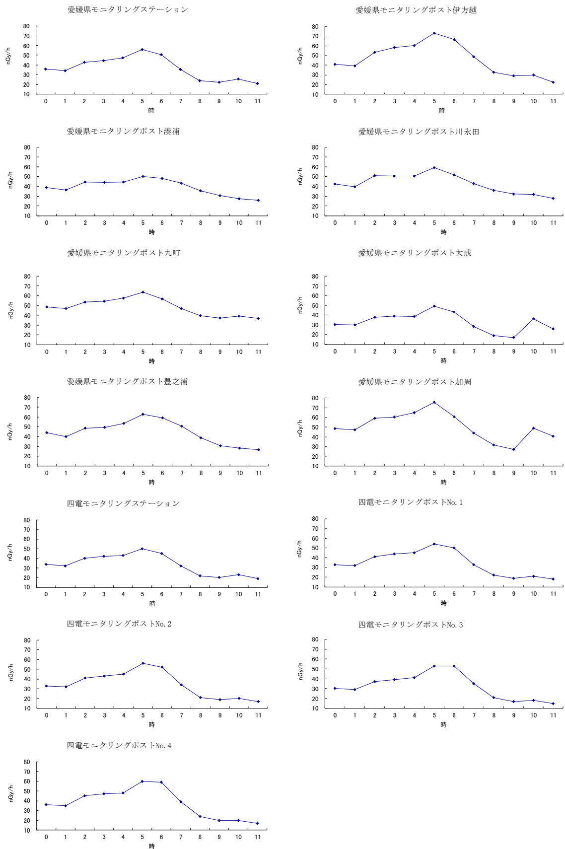
図 13 異なる方位のモニタに同時に発生している例（1 時間平均値） (NaI(Tl)シンチレーション検出器)（令和 3 年 8 月 15 日）
