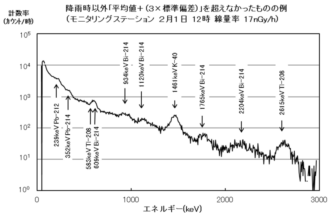
図9 愛媛県測定局 (NaI (Tl) シンチレーション検出器) における 空間ガンマ線スペクトル図 (降雨時以外の例)
